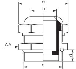
Metal Rakorlar PG ve METRİK
